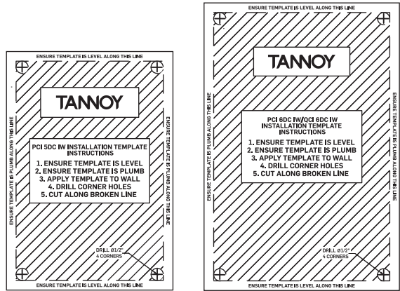
Fig. 1.Cutout Templates
