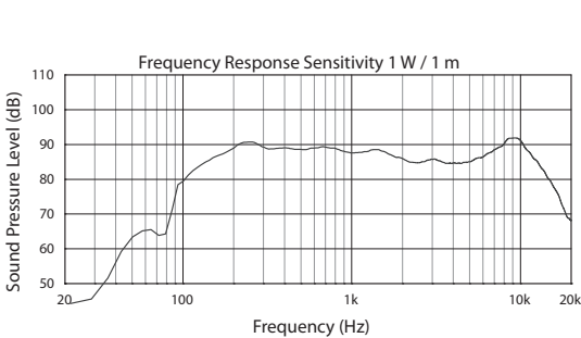
Graph 1# VLS 7 (EN 54)
