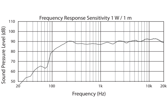
Graph 2# VLS 15 (EN 54)
