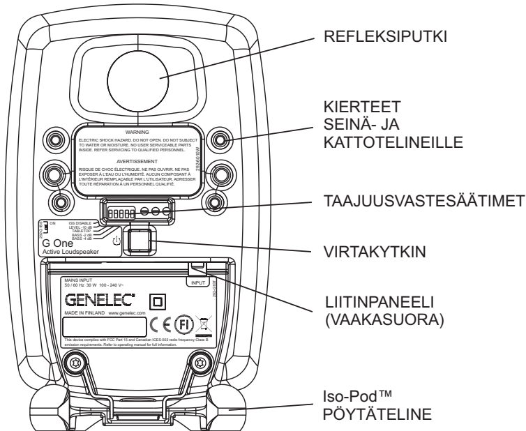
Kuva 1. G One:n liitännät ja säätimet.
