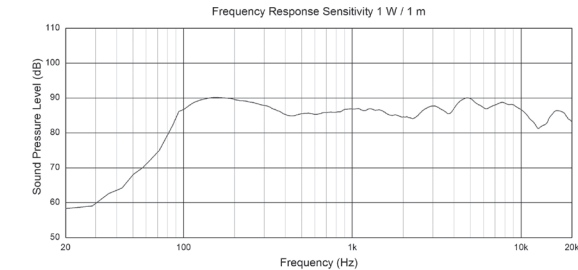
Graph 2# CVS 4 (EN 54)_01_SPL
