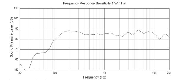
Graph 3# CVS 4 MICRO (EN 54)_01_SPL
