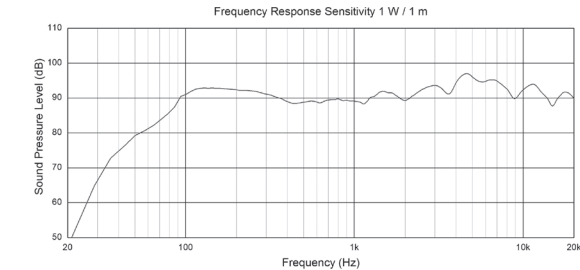
Graph 1# CVS 6 (EN 54)_01_SPL
