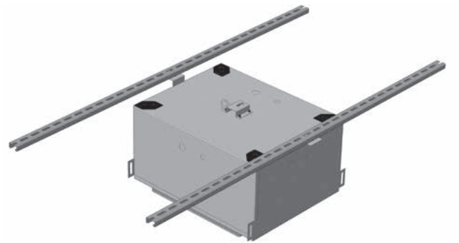
Rückendose zwischen Schienen montiert
