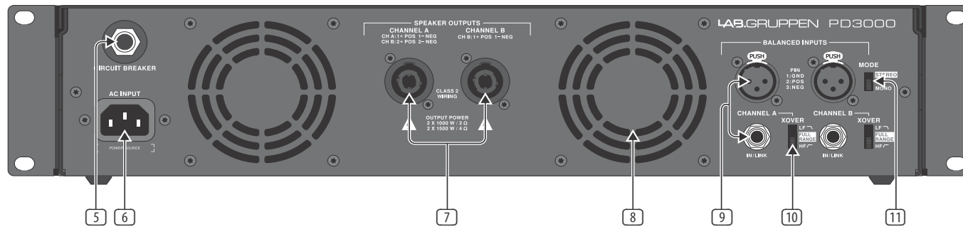
Afb. 2: PD3000 Achterpaneel
