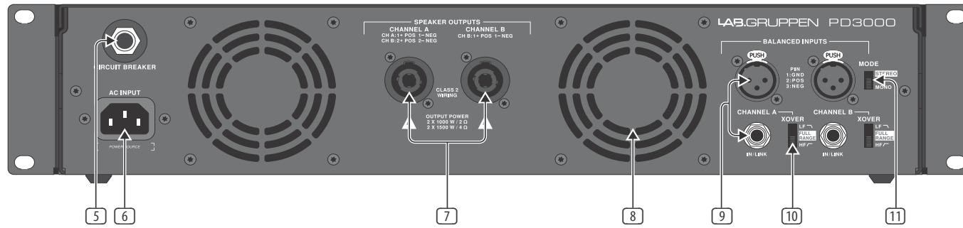
Fig. 2: Pannello posteriore del PD3000
