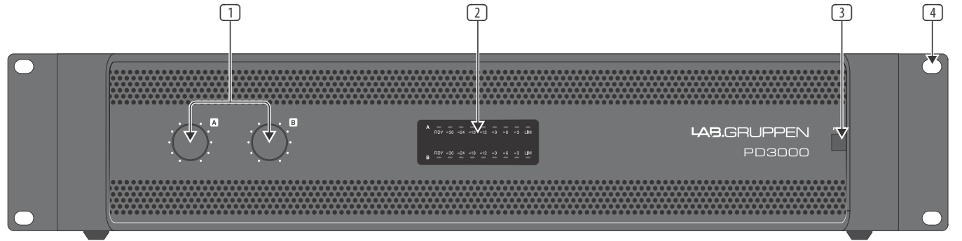
Bild 1: PD3000 frontpanel
