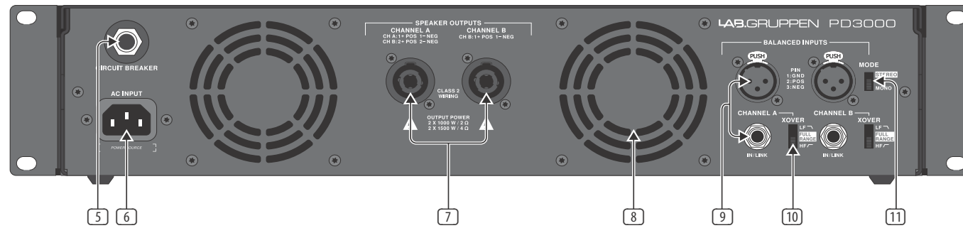
Rys. 2: Tylny panel PD3000
