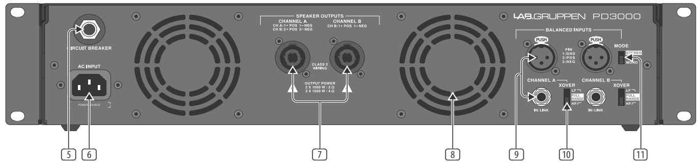
Bild 2: PD3000 bakpanel
