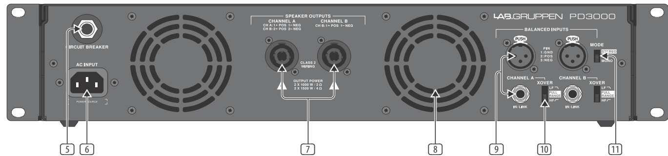
Fig. 2 : Panneau arrière du PD3000
